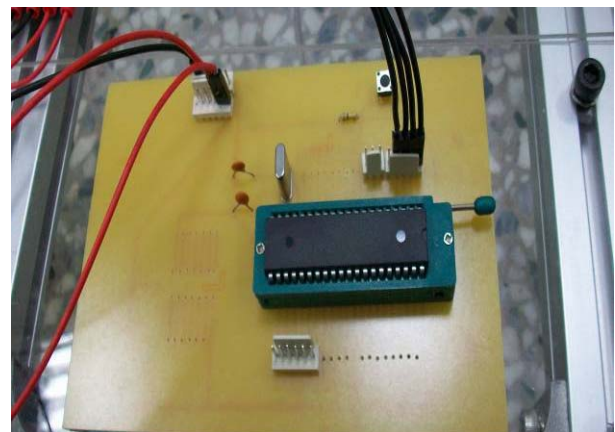
圖八、8051 電路圖設計實體圖
