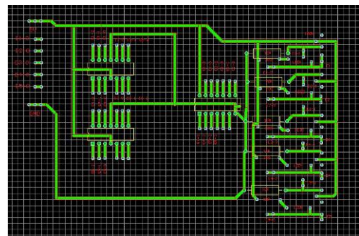
圖九、感測器電路佈線圖
