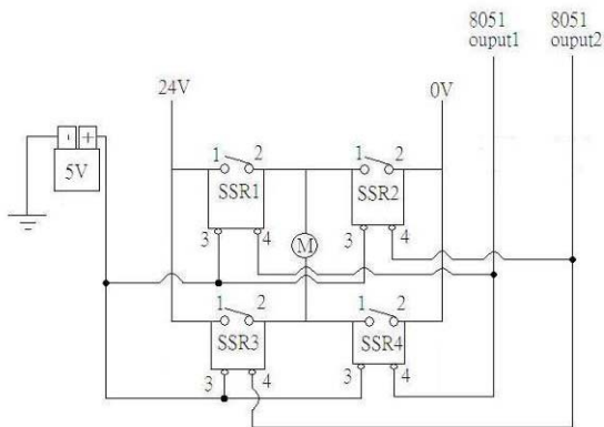
圖五、馬達正反轉電路圖
