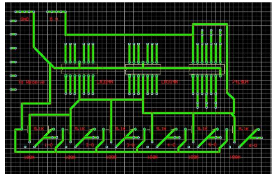
圖十三、紅外線處理板電路佈線圖
