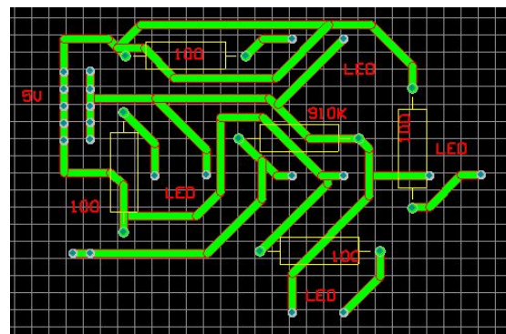
圖十五、紅外線訊號電路佈線圖
