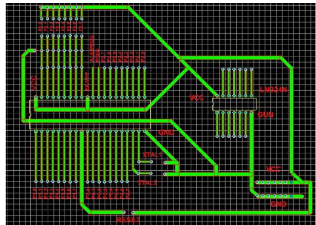
圖七、控制電路佈線圖
