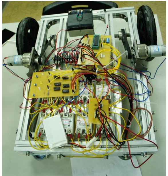
圖三、底盤電路
