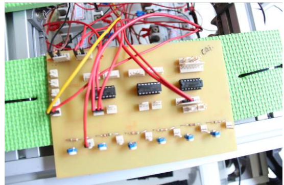
圖十四、紅外線處理板實體圖
