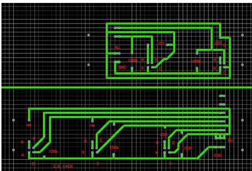
圖十一、CNY70 電路佈線圖
