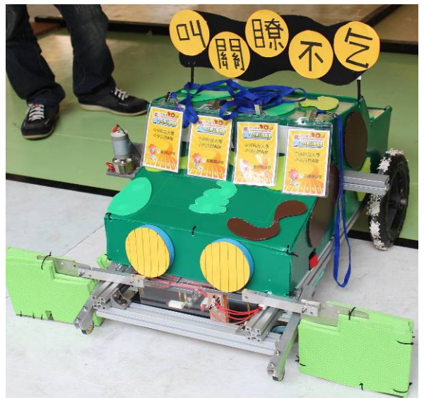
圖四、左右兩側為踢球機構
