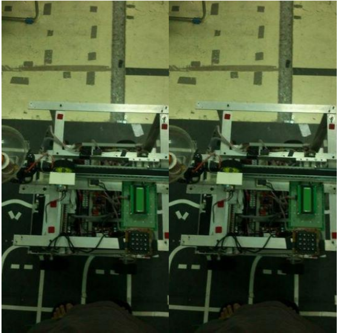
說明：前方裝有夾取聖杯之夾爪。
