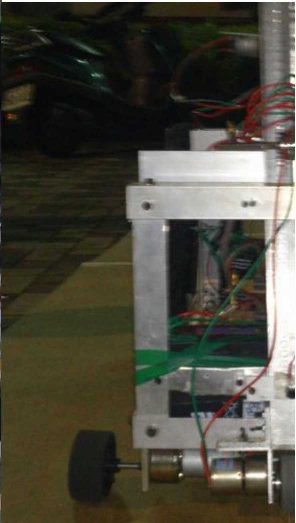
說明：支撐和動力裝置，能順利跨越 30 公分階梯。
