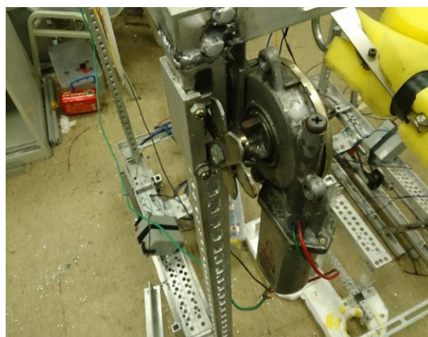
圖 10 機器人升降機構
