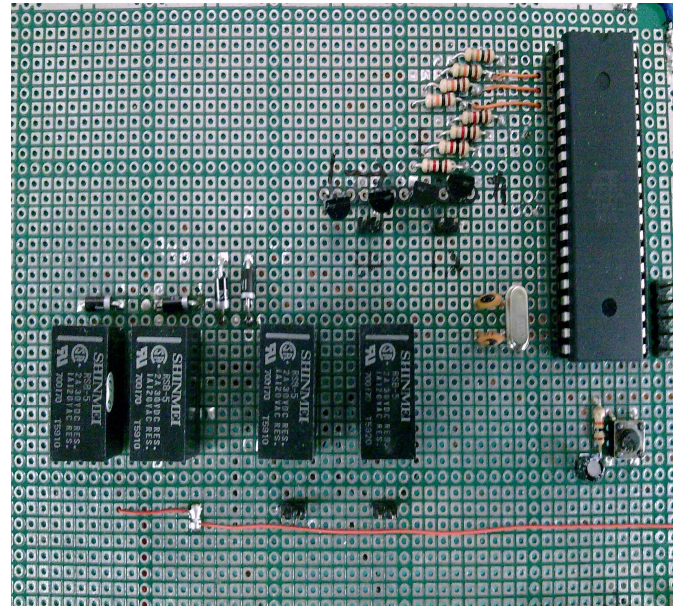
8051 控制板
