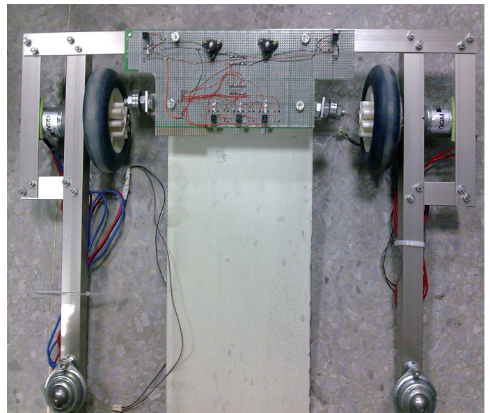
底盤
