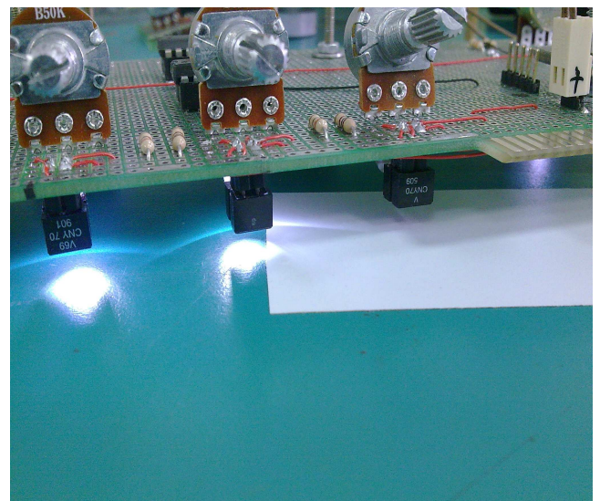
CNY70 感測器
