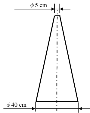
圖四 五專及二專組競賽項目二，龍王及小龍示意圖
